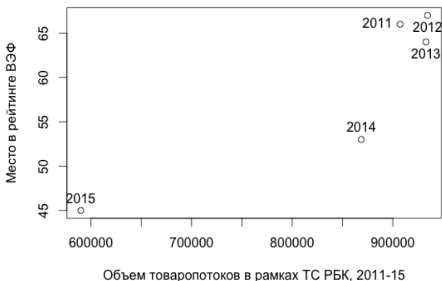
Рис. 1. Диаграмма рассеивания
